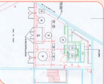
A: Caseta mescladora / B: Tanq Nitrogen / C: Pulmó de mesclador / D: Tanq Oxigen / E: Gasificador d'oxigen / F: Gasificador de nitrogen / G: Blocs d'ampolles / H: Central de reserva de 10-10 / I: 1000 m 3 cúbics / K: Pumpes.
