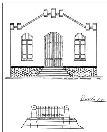
Dibuix fet per Celestí Bellera del nou grup escolar de Palou, c. 1922. Font: AMGr, Fons Celestí Bellera i Rita Gibernau.
