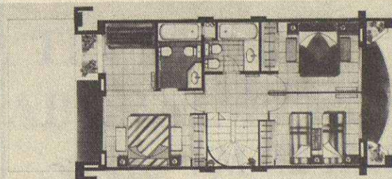
P. PISO
