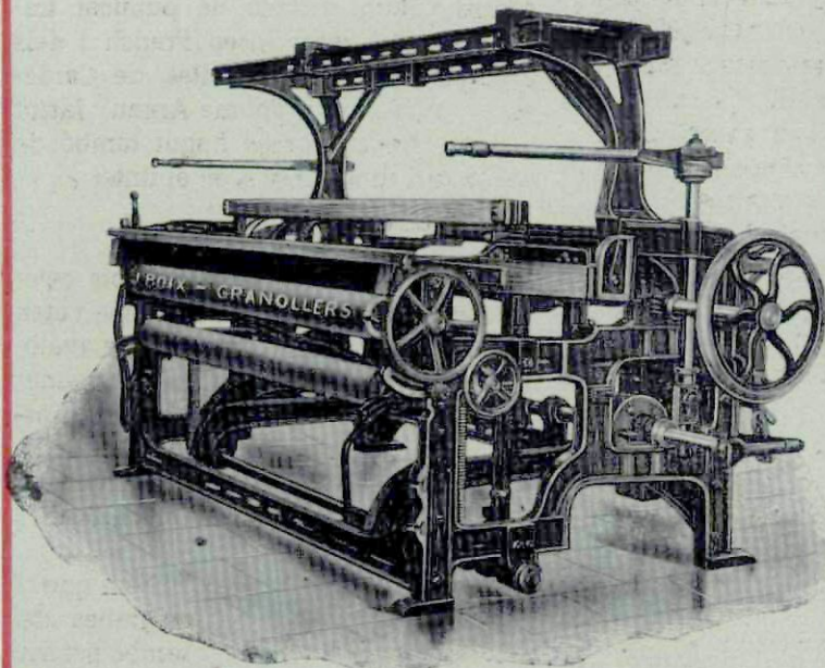
Teler amb doble pont, especial per a teixits de seda, llana i cotó
