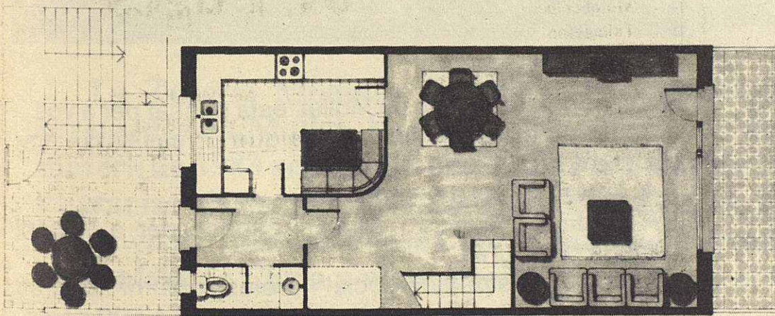
PLANTA 1º PISO ( SUP APROX. 63.00 m 2 + 21.00 m 2 terraza )
