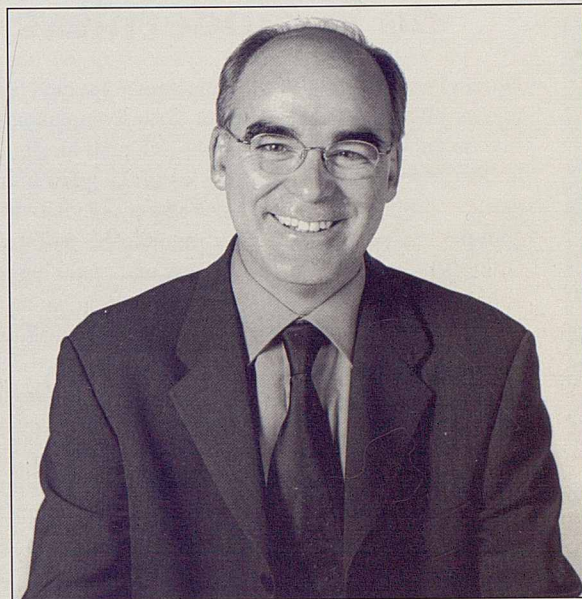
Foto: Jordi Ribó (HMG)
