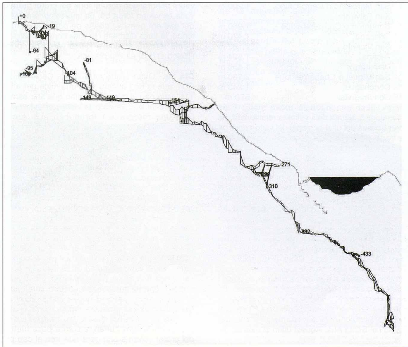
ESQUEMA TOPOGRÀFIC DE L'ALÇAT DEL SISTEMA BARGADERA
