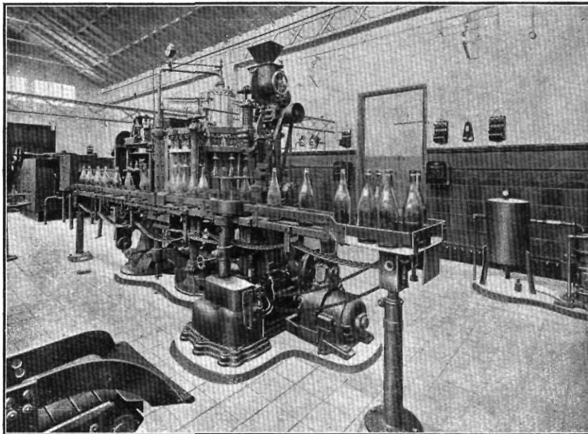
Tren automàtic per a embotellar, mogut per electricitat i aire comprimit
