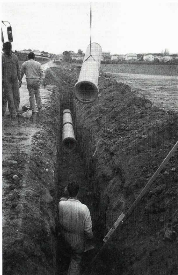
Col·lector general d'aigües residuals al camí de Bonaire.
