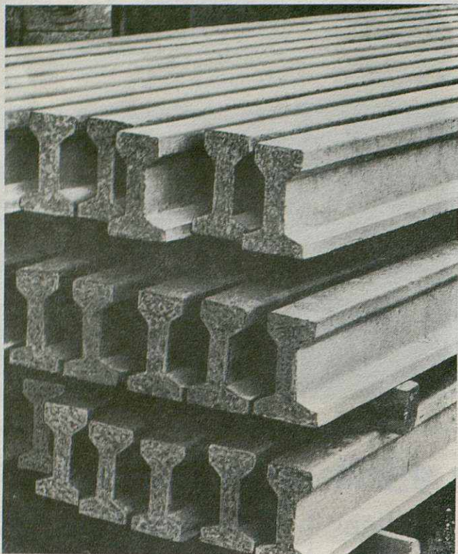
VIGUETA PRETENSADA AUTORRESISTENTE DE 16 cms.
