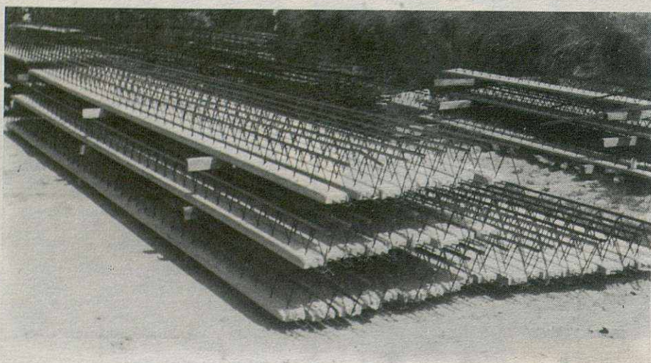
SEMIVIGUETA ARMADA TIPO D. C.
