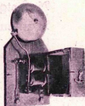
Timbres elèctrics
