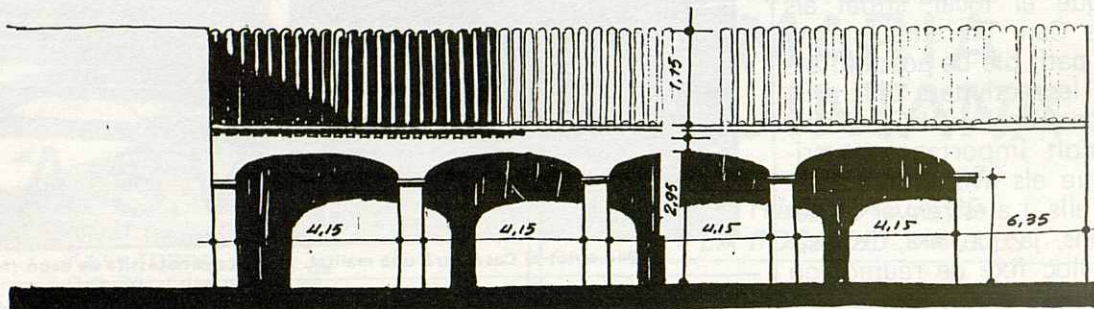
ALZADO.
